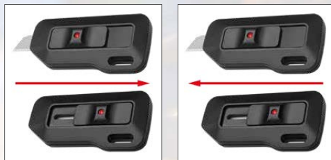
automatischer Klingentrückzug durch federbelastete Klinge
